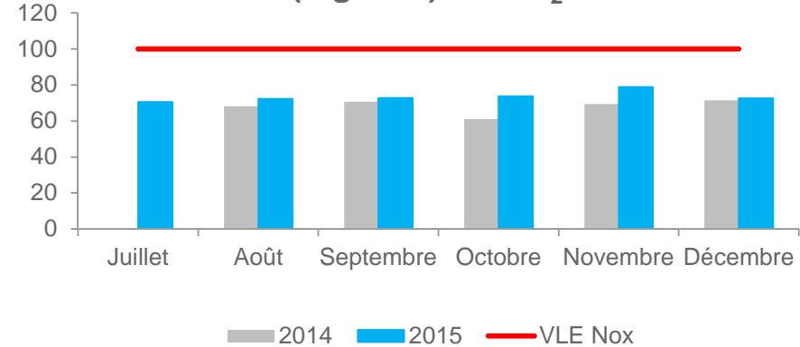
Concentration moyenne mensuelle en NOx (mg/Nm 3 ) à 3%O 2
